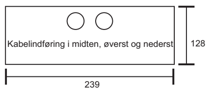
Udskæringsmål IB6
